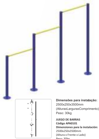
JOGO DE BARRAS Código APA0101
